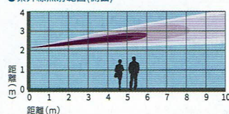
●紫外線照射範囲(側面)
