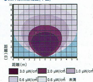
●紫外線照射範囲(平面)
